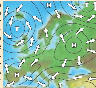
Europakarte mit Hoch- (H) und Tiefdruckgebieten (T). Der Wind (Pfeile) fließt von den Hoch- zu den Tiefdruckgebieten und dreht dabei im (H) und gegen den Uhrzeigersinn (T).
